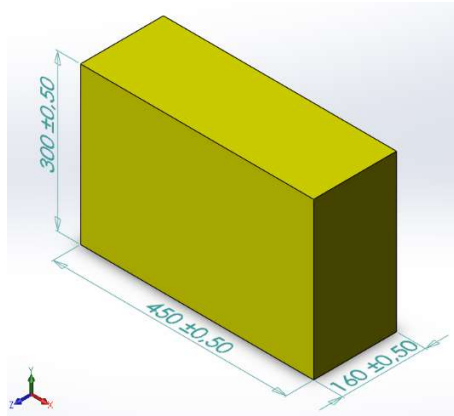
Şekil-13 Görev 2 Sarı Kutu Malzemesi Ölçüleri
