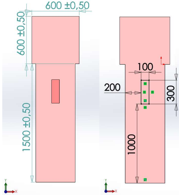
Şekil-20 Gökbeğlítepenin İçerisinde Bulunan T Sütunu Ölçüleri
